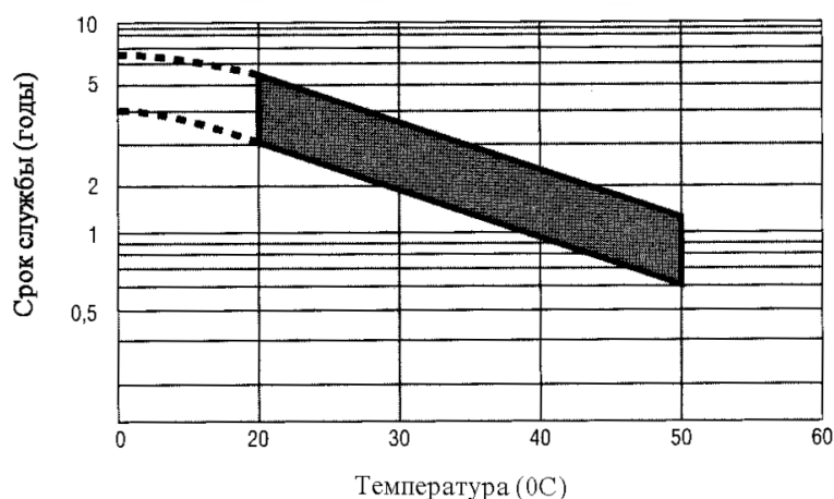
Рисунок 13– Срок службы при буферном режиме использования батареи
