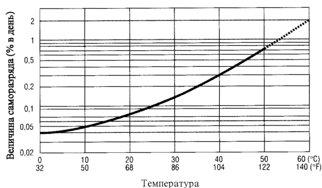
Рисунок 6 – Зависимость величины саморазряда от температуры
