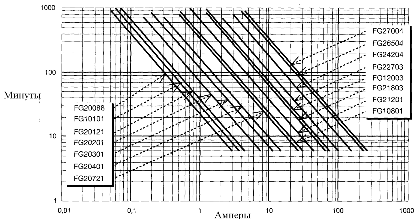
Рисунок 16 – Выбор аккумулятора требуемой мощности
