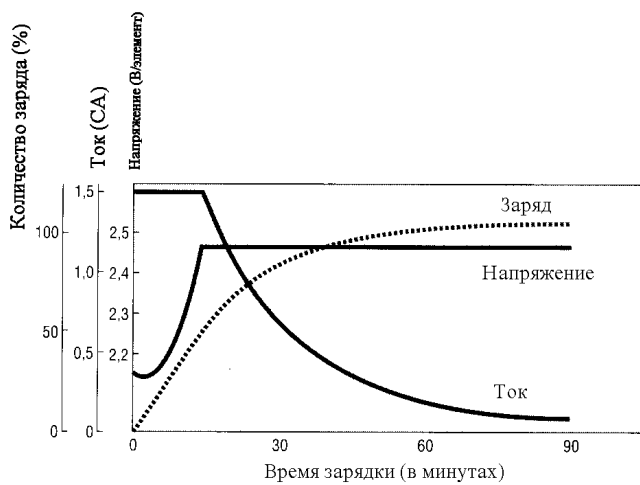
Рисунок 10 – Характеристики быстрой зарядки батареи Батарея: 70% - зарядка Температура: 25°C (77°F)
