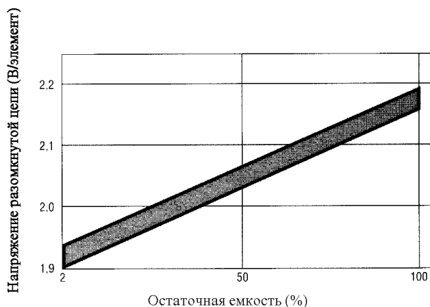
Рисунок 7 – Зависимость между напряжением разомкнутой цепи и остаточной емкостью батареи
