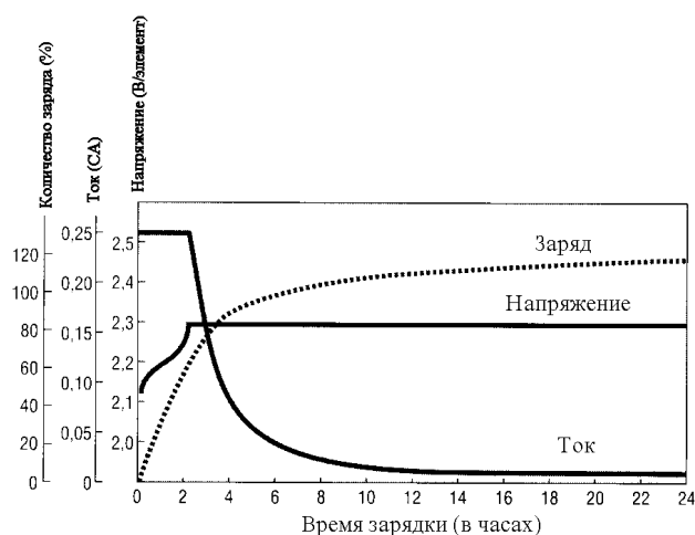
Рисунок 9 – Характеристики заряда при постоянном напряжении (2.30В/элемент, 25°С (77°F))
