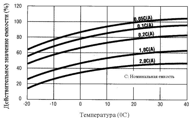
Рисунок 4 Зависимость емкости от температуры
