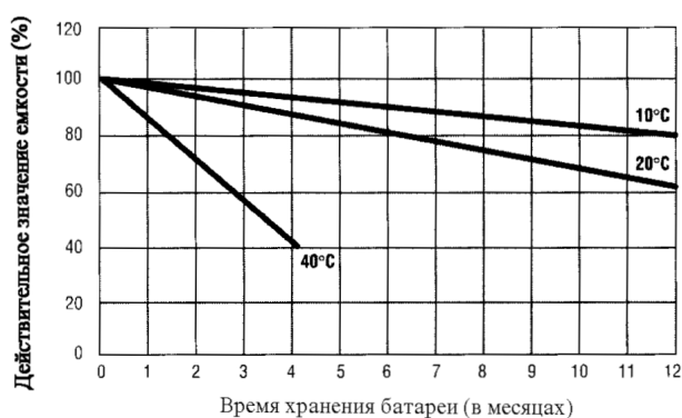
Рисунок 5 – Величина саморазряда
