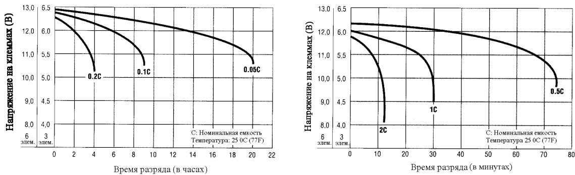
Рисунок 3 – Зависимость времени разряда от тока разряда
