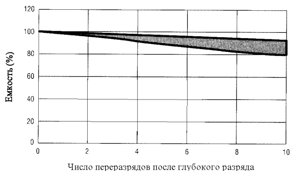
Рисунок 14 – Зависимость между числом перезарядов и действительной емкостью батарей (в процентах от номинальной)
