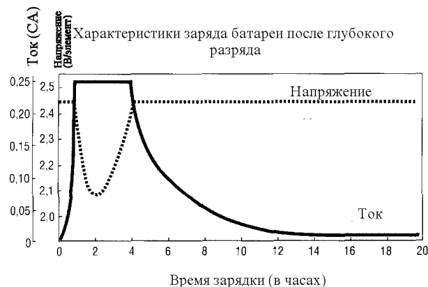
Рисунок 15 – Характеристики заряда батарей после глубокого разряда
