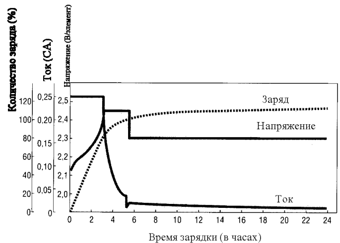
Рисунок 11 – Двухступенчатый заряд батареи 2.45 В/элемент и батареи 2.30 В/элемент при 25°C (77°F)
