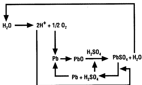
Рисунок 2 Рекомбинационный цикл
