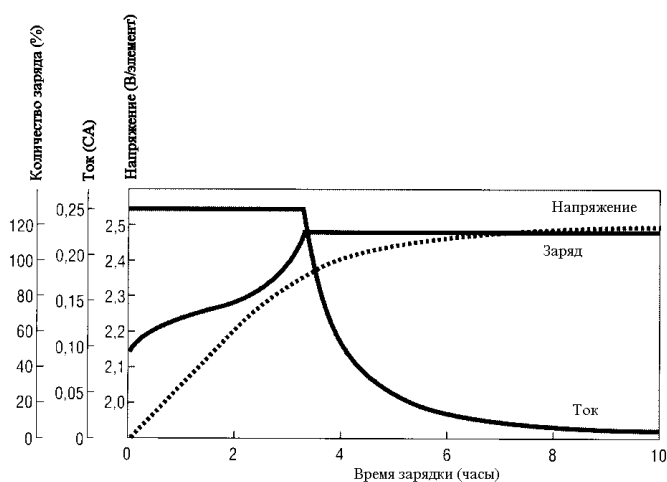
Рисунок 8 – Характеристики заряда при постоянном напряжении (2.45В/элемент, 25°С (77°F))
