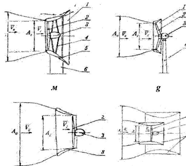
Рис. 15. Схемы горизонтально-осевых ветродвигателей с воздуховодными устройствами:
