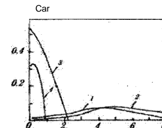
Рис. 14. Зависимость коэффициента крутящего момента C_m от коэффициента быстроходности X :
