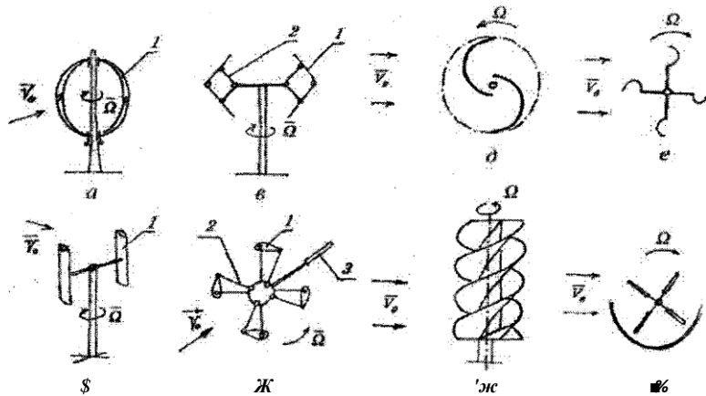
Рис. 7. Ортогональные вертикально-осевые ветродвигатели: а - ротор Дарье; б - ротор Н-типа; в - ротор Масгроува (в полусложенном положении) с изменяемым положением лопастей; г - ротор «жиромилл» (вид сверху) с изменяемым углом установки лопастей; д - ротор Савонцуса (вид сверху); е — ротор чашечный (анемометр, вид сверху); ж - ротор шнековый; з - ротор пластинчатый с экраном, карусельный (вид сверху); 1 - лопасть, 2 - механизм управления положения лопастей; 3 - флюгер
