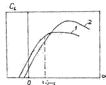
Рис. 19. Зависимость коэффициента подъемной силы C_L от угла атаки \alpha : 1 - профиль, используемый для регулирования срывом потока; 2 - традиционный крыловой профиль
