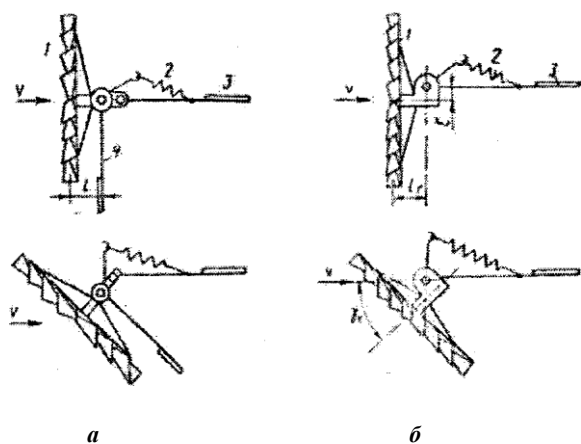
Рис* 20. Схема регулирования ветродвигателя выводом из-под ветра: а - при помощи боковой поверхности; б - за счет эксцентриситета; 1 - ветроколесо; 2 - пружина; 3 - флюгер; 4 - боковая поверхность
