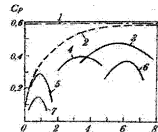
Рис. 13. Зависимость коэффициента использования энергии ветра C_p от коэффициента быстроходности X :
