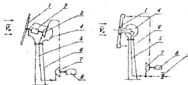
Рис 11. Схемы пневматической передачи: а - с компрессором
