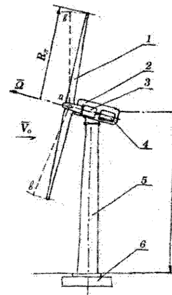
Рис. 1. Конструктивная схема горизонтально-осевого ветроагрегата: 1 — ветродвигатель; 2 - гондола; 3 - мультипликатор; 4 - нагрузка (электрогенератор); 5 - башня; 6 - фундамент
