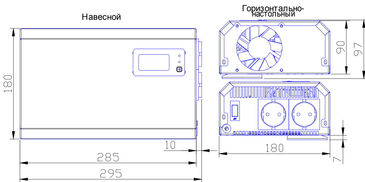
б) ИнСтаб 1000; ИнСтаб 1500
