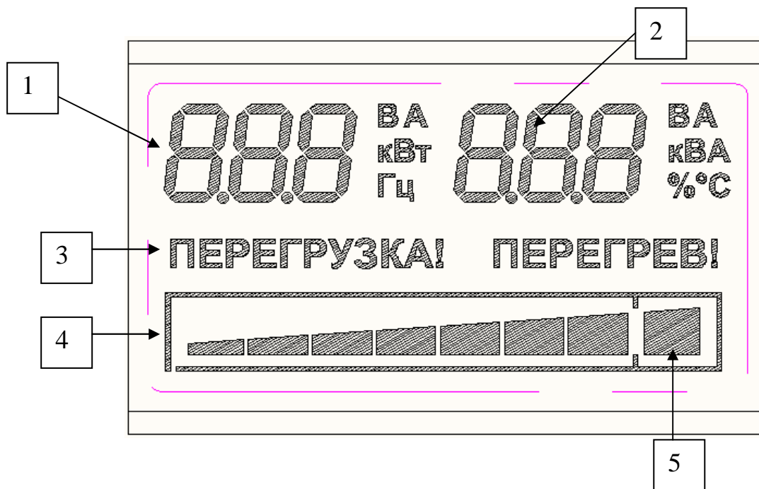
Рисунок 3 – ЖК-дисплей (для моделей ИнСтаб 1000, ИнСтаб 1500, ИнСтаб 3500)
