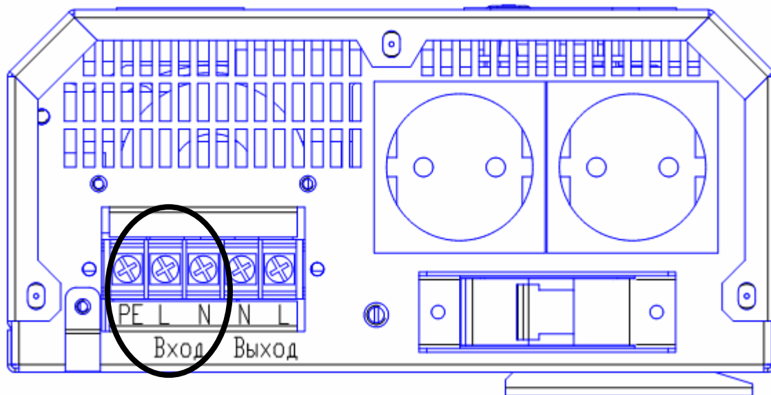
Рисунок 3.2 – Стабилизатор ИнСтаб 3500.
