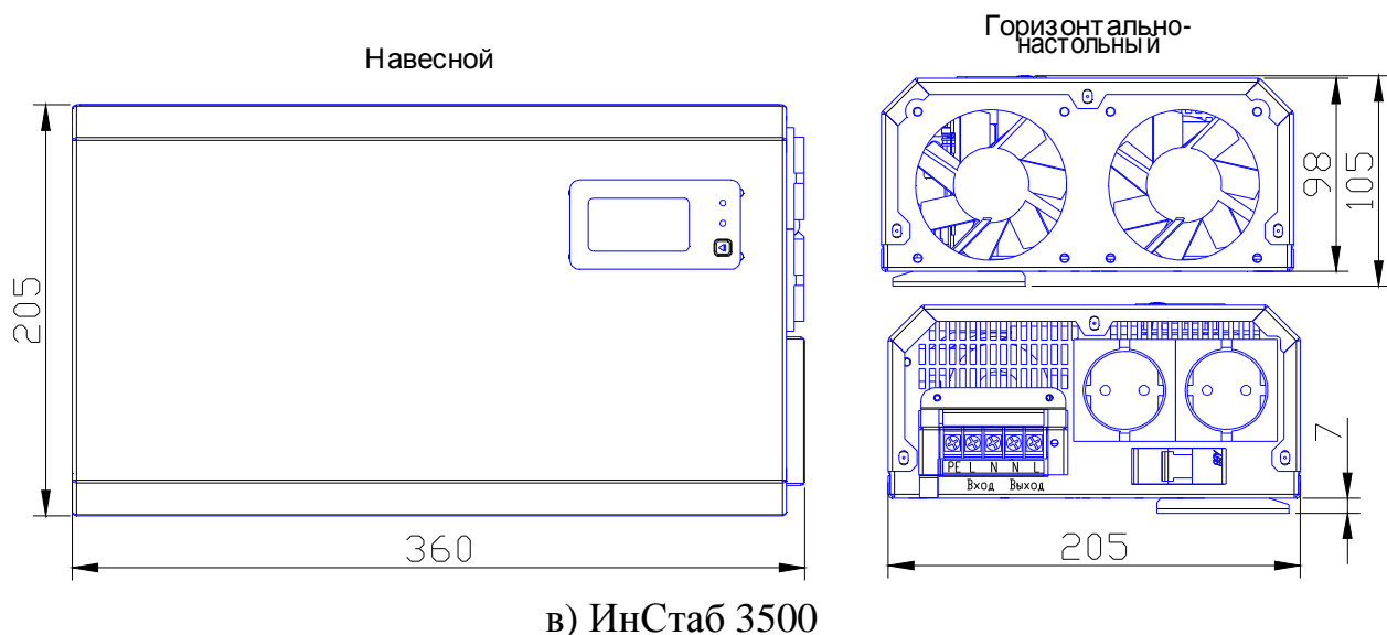
Рисунок 1.2. – Габаритные размеры стабилизатора Штиль и рекомендованные варианты установки а) ИнСтаб 500; б) ИнСтаб 1000; ИнСтаб 1500; в) ИнСтаб 3500
