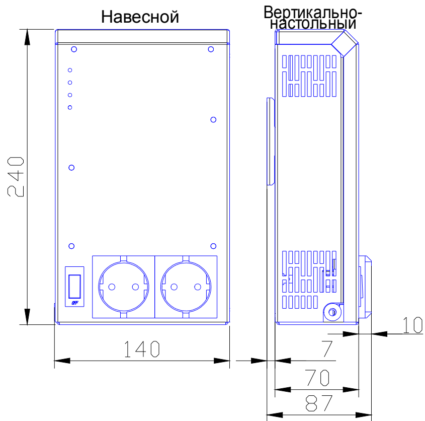
а) ИнСтаб 500
