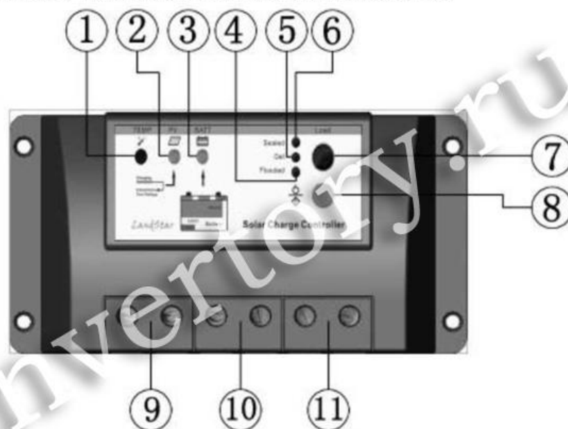
Рис. 2.1. Элементы управления и индикации контроллера
