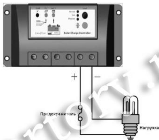
Рис. 3.3. Подключение нагрузки
