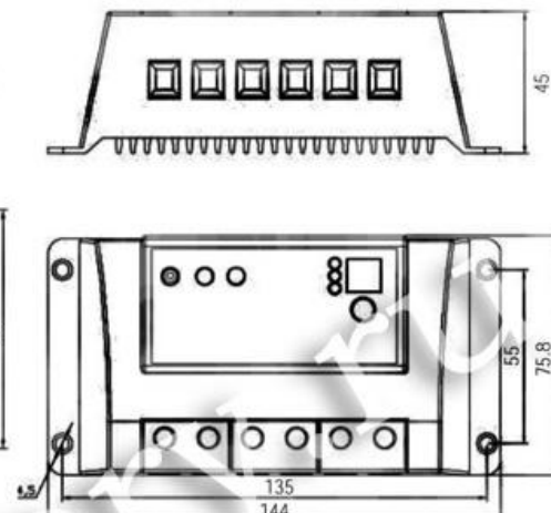
Модели LS1524 и LS2024
