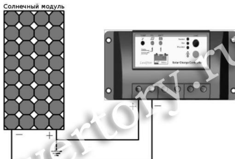
Рис. 3.4. Подключение ФЭМ
