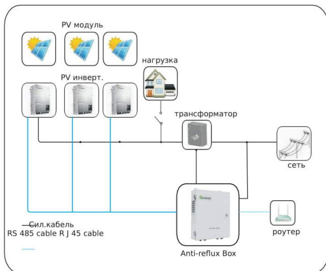
1-фазная система
