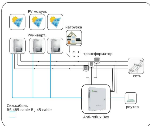
3-фазная система
