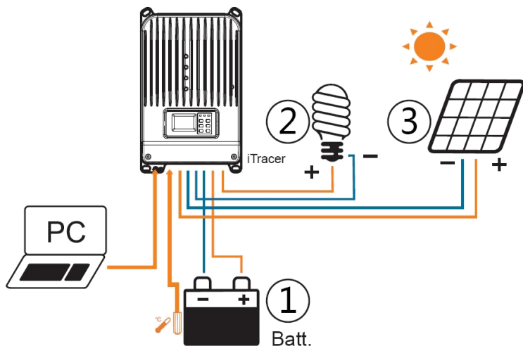
Соединение
